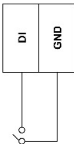
DI Dry Contact
