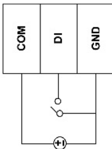
DI Wet Contact
